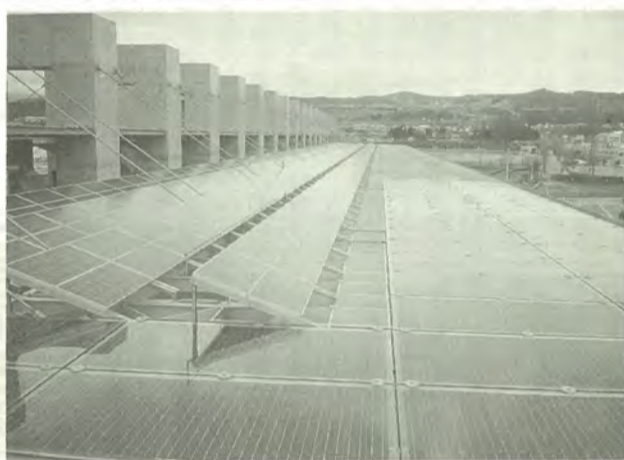
ハイテクプラザ会津若松技術支援センター建設 太陽光発電工事(会津若松市一箕町)
